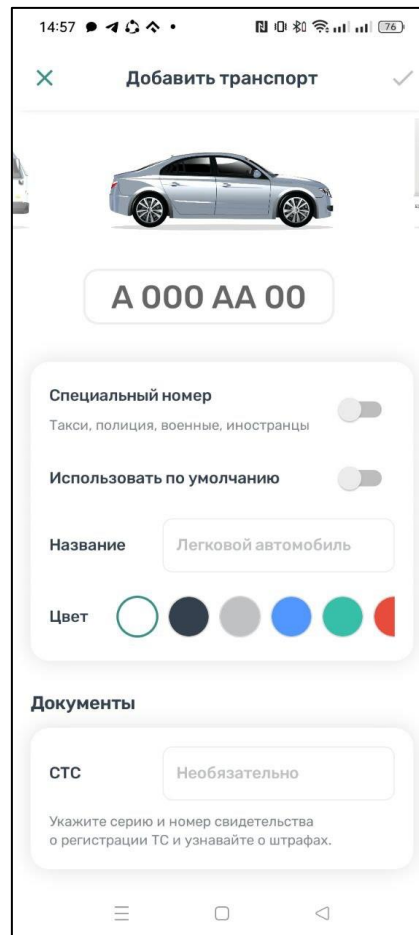
Рисунок 39 – Добавление ТС
