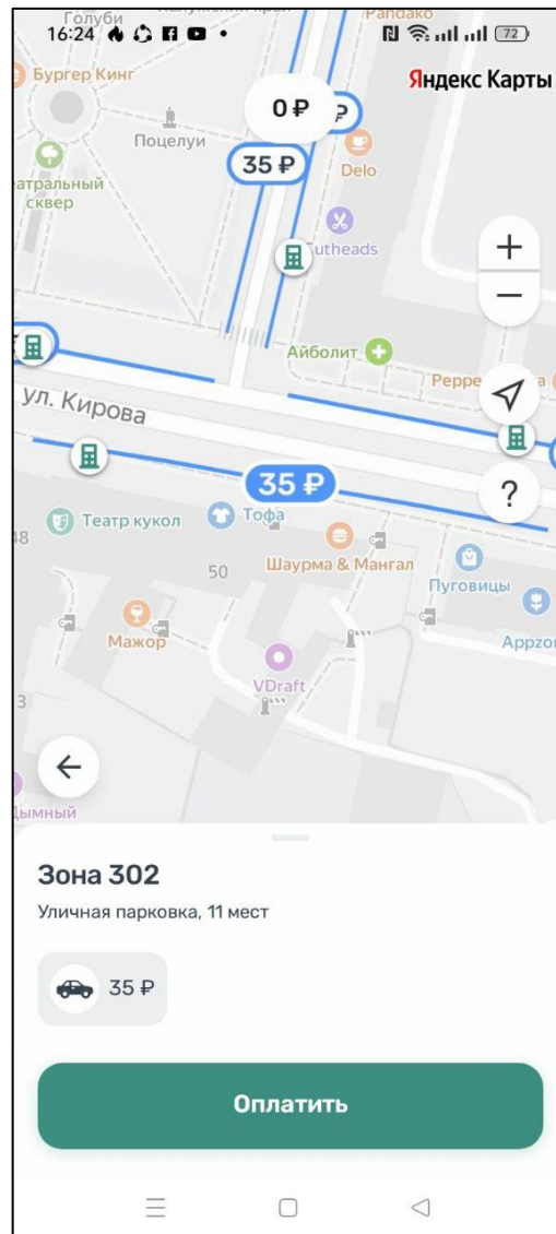
Рисунок 30 - Оплата парковки
