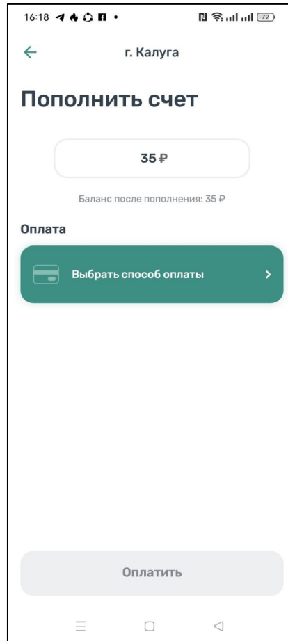
Рисунок 23 - Пополнить счет
