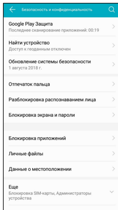
Рисунок 17 - Настройки Android
