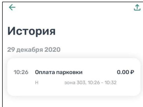
Рисунок 29 – История операций
