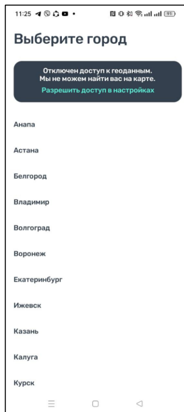
Рисунок 4 – Выбор города
