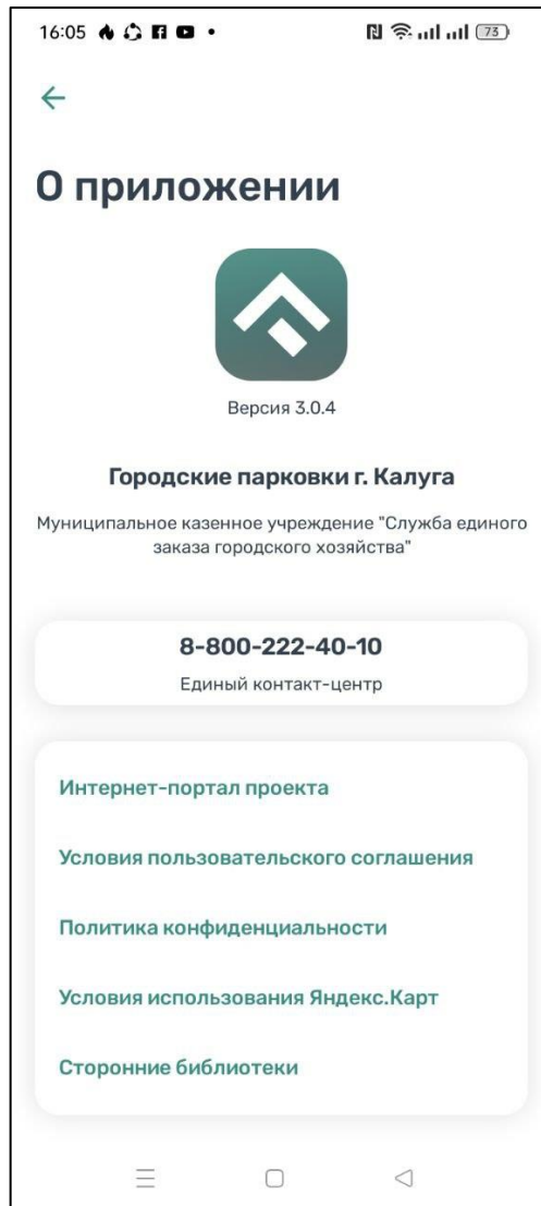
Рисунок 20 – Справочная информация
