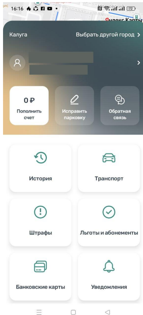
Рисунок 21 – Меню приложения
