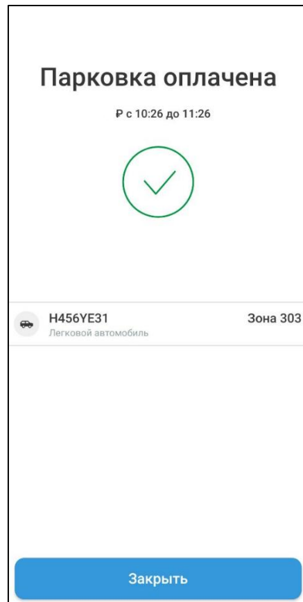
Рисунок 32 – Оплата парковки
