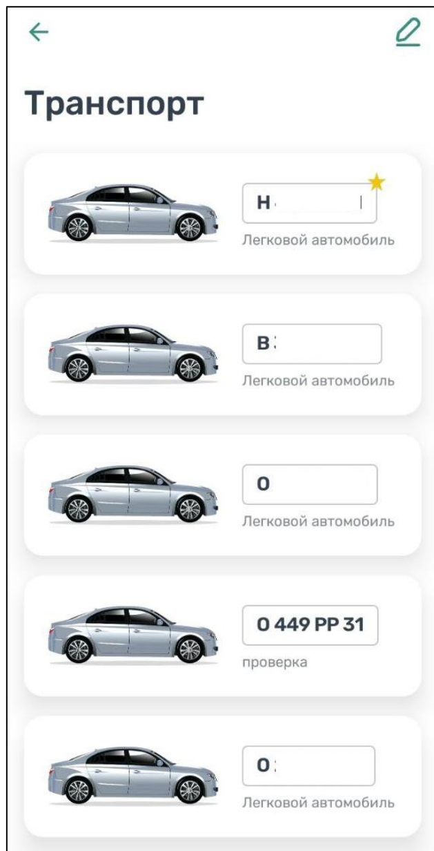
Рисунок 38 – Список ТС
