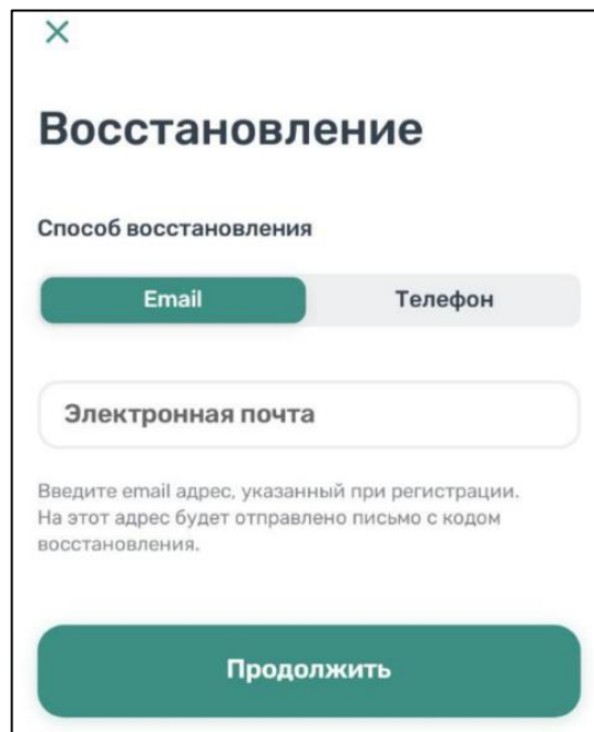
Рисунок 15 - Восстановление пароля
