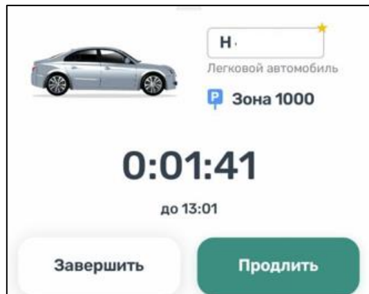
Рисунок 33 – Текущая парковка
