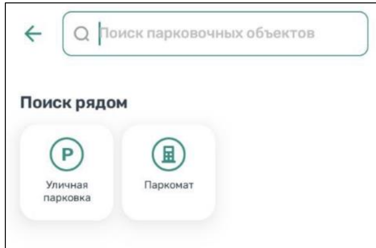
Рисунок 18 – Выбор объекта
