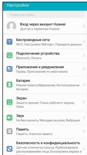
Рисунок 16 - Настройки Android
